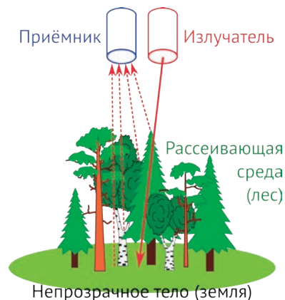
Рис. 3.3 Принцип действия Lidar
