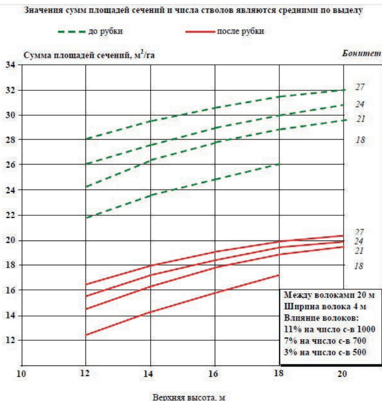
Рис. 2.22 Графические модели рубок ухода для сосняков Южной Финляндии [46]
