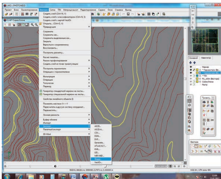
Рис. 3.16 Программа PHOTOMOD [123]
