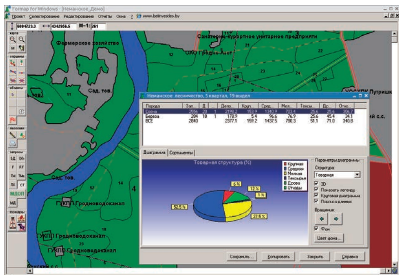
Рис. 3.12 ГИС-программа Formap [113]
