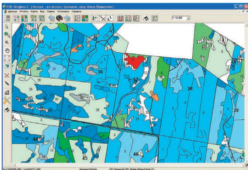
Рис. 3.11 ГИС-программа «Лесфонд» [112]
