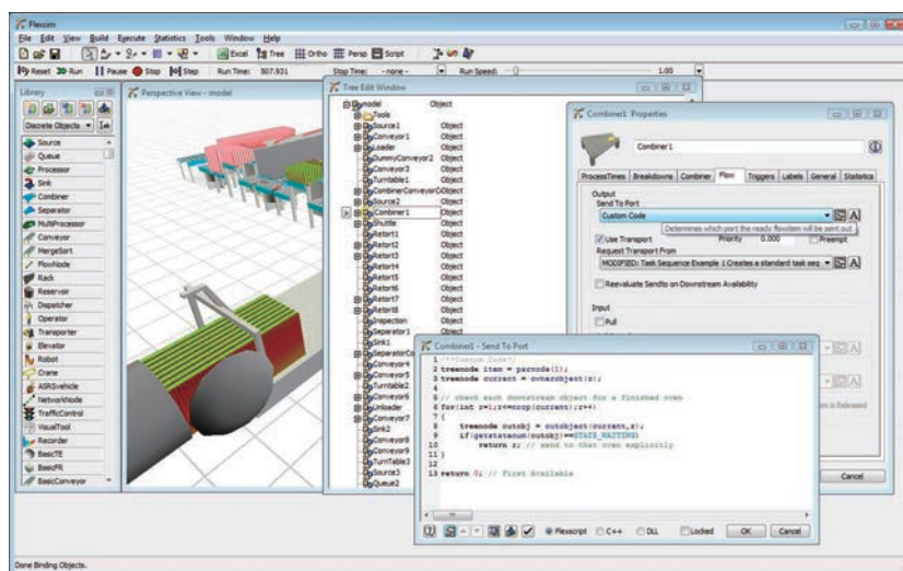
Рис. 3.19 Пример интерфейса Flexsim [130]
